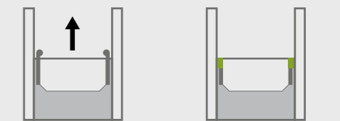
Der Butyl Dichtstoff bewegt sich in den sichtbaren Scheibenzwischenraum.
